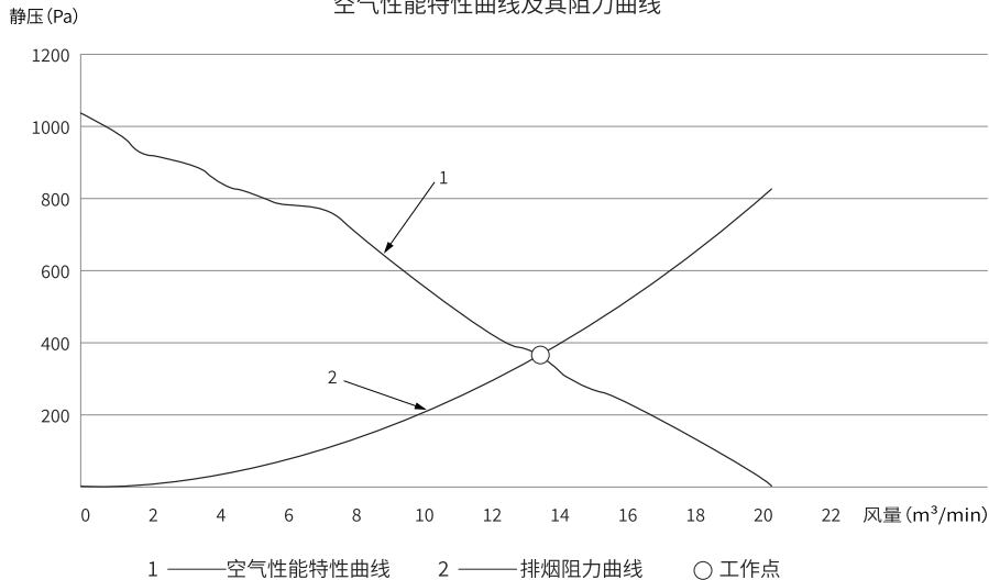
空气性能特性曲线及其阻力曲线
