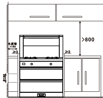
图二、产品尺寸图 单位 mm
